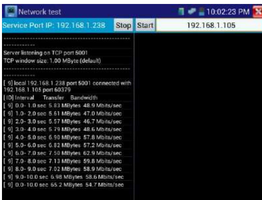
Рис. 3.3.27-4 Запуск сервера
