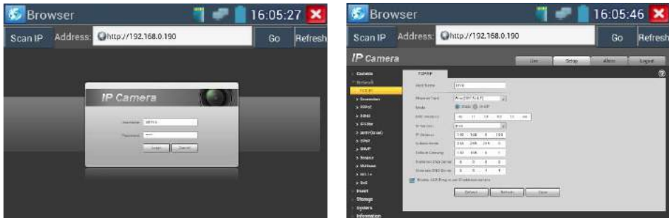
Рис.3.3.24-1 Встроенный браузер
