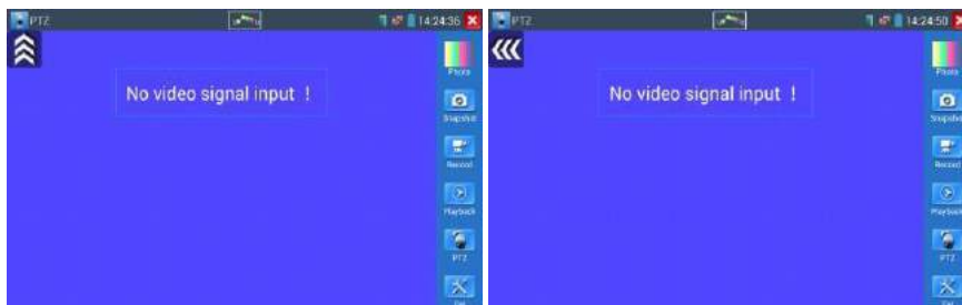
Рис.3.3.1-3 Управление движением
