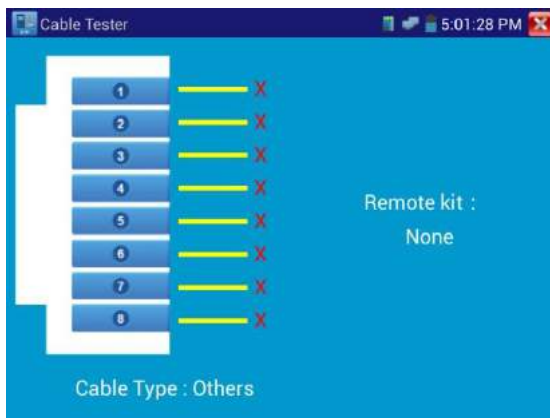
Рис. 3.3.11-1 Тестер кабеля
