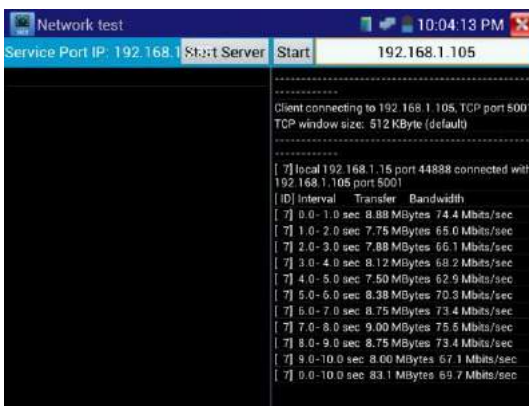
Рис.3.3.27-5 Запуск клиента
