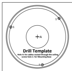
Рисунок 2-4 Шаблон крепления
