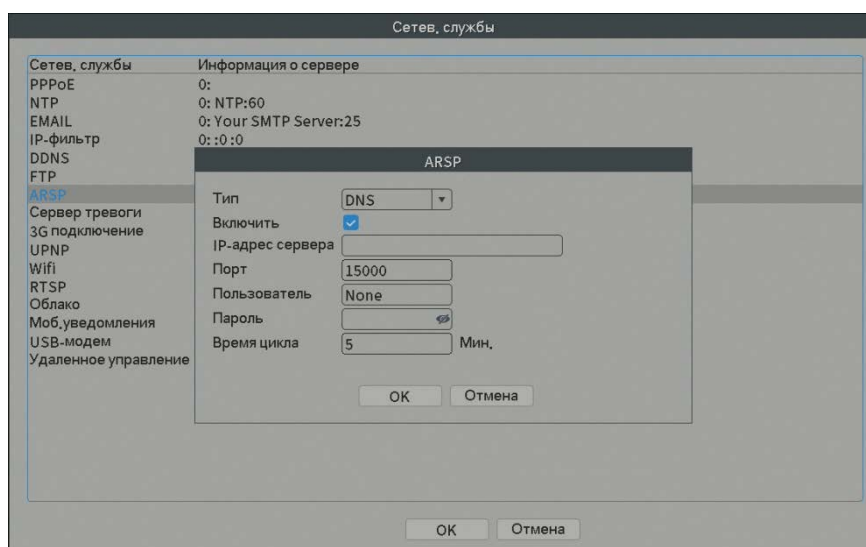
Рис.4.31 ARSP-сервер
