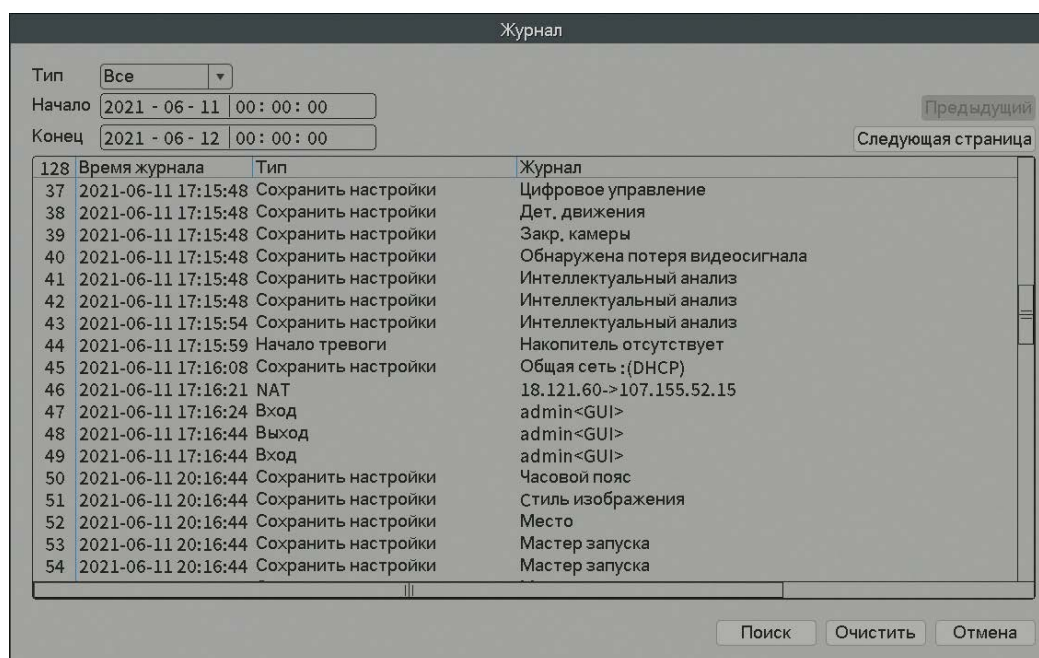
Рис.4.21 Информация системного журнала
