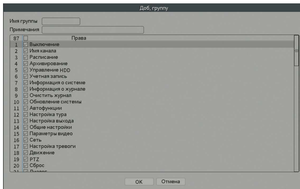
Рис.4.49 Добавление группы
