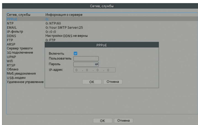
Рис.4.25 Настройки PPPoE
