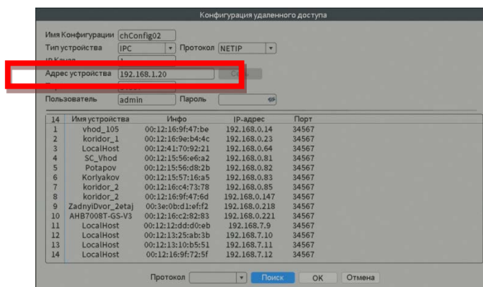
Рис.4.15 Поиск камер
