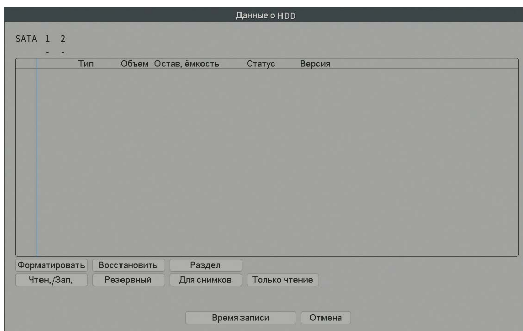
Рис.4.19 HDD информация
