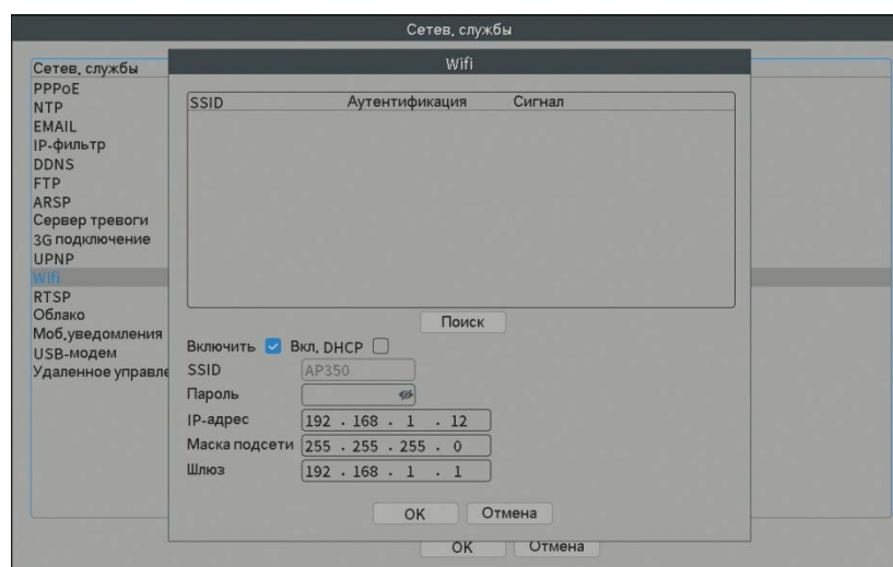
Рис.4.35 Wi-Fi
