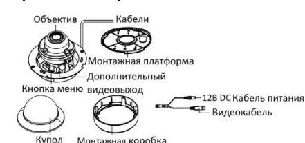
Рисунок 1-13 Купольная камера III типа
