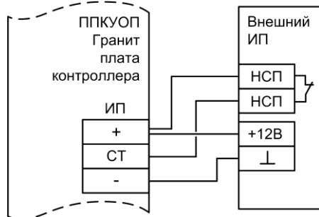
Рис.Б6 Схема подключения внешнего источника электропитания (ИП)
