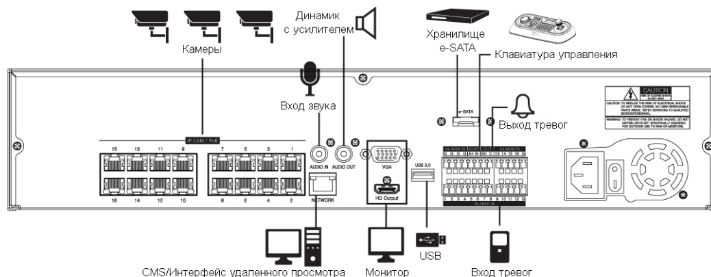
Рис. 2-1 Порядок подключения
