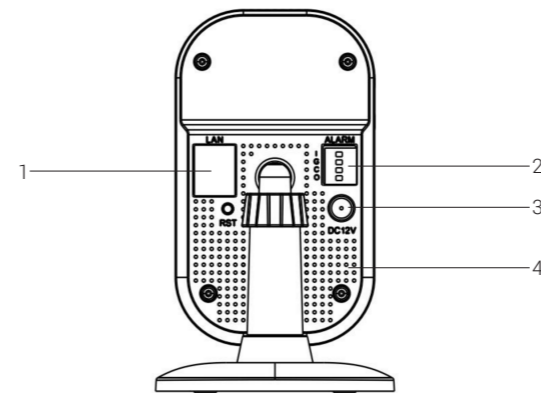
Рисунок 1 Разъемы видеокamеры
