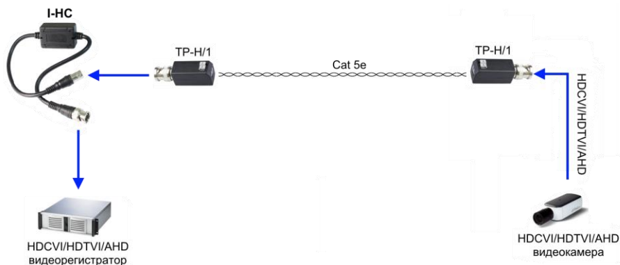
Рис.4 Типовая схема подключения изолятора I-NC через кабель витой пары с использованием приемопередатчиков TP-H/1
