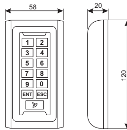
Рис.1 Габариты и крепежные отверстия
