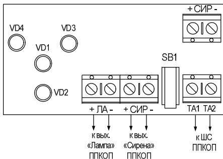
Рис. 2 Схема подключения оповещателя
