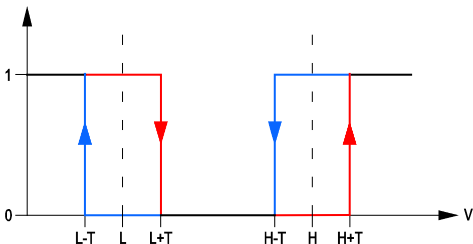
Рис. 10. Способ работы аналогового входа. 0 – отсутствие нарушения. 1 – нарушение. L-T – уровень напряжения L минус допустимое отклонение. L – нижний уровень напряжения. L+T. L+T – уровень напряжения L плюс допустимое отклонение. H-T - уровень напряжения H минус допустимое отклонение. H – верхний уровень напряжения. H+T – уровень напряжения H плюс допустимое отклонение.
