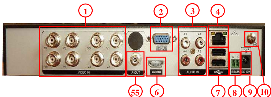
Задняя панель:
