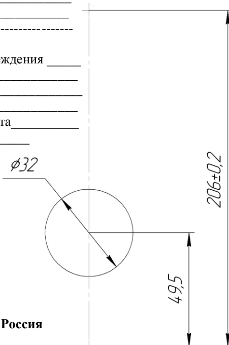
Рис. 1. Разметка под установку блока вызова
