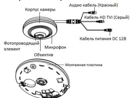
Рисунок 1-26 Панорамная камера
