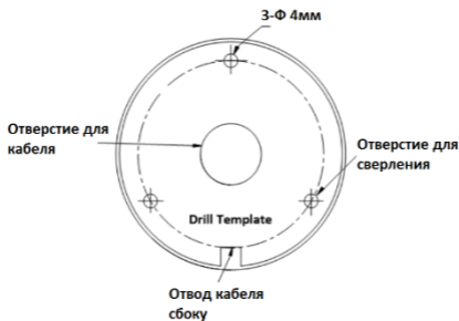
Рисунок 2-1 Шаблон крепления
