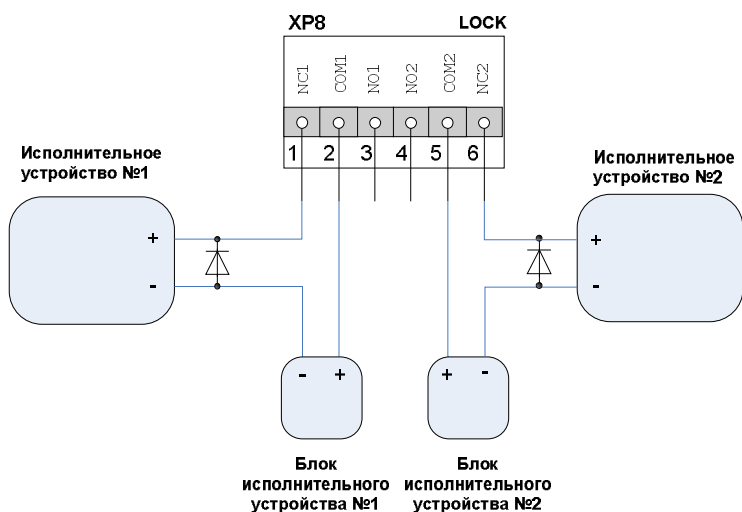
рис. 9. Схема подключения электромагнитных замков при двухдверном режиме работы контроллера
