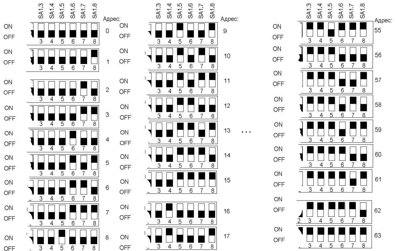
рис. 26. Примеры установки сетевых адресов при помощи DIP-переключателя SA1.
