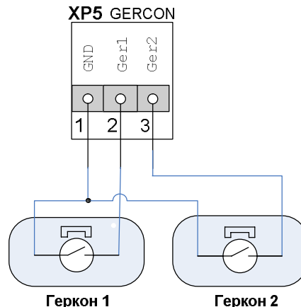
рис. 13. Разъем XP5 (GERCON) с примером подключения герконов
