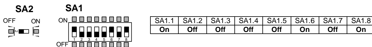
рис. 23. Пример установки сетевого адреса «05» и скорости обмена 57600 бит/с для контроллера, не последнего в сети с однодверной конфигурацией
