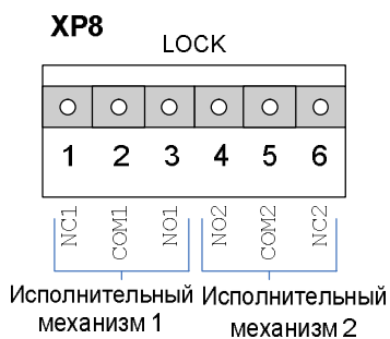
рис. 6. Разъем XP8 (LOCK)
