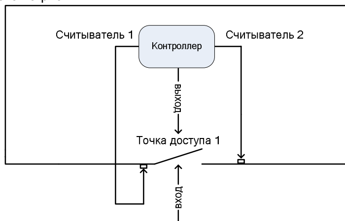
рис. 4. Пример работы контроллера в ододверном режиме работы с функцией АРВ
