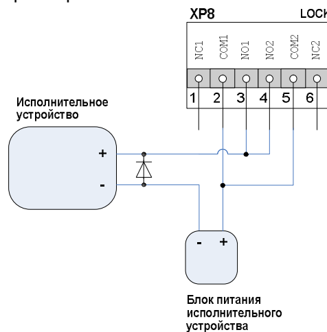
рис. 8. Схема подключения электромеханических замков при однодверном режиме работы контроллера через контакты обоих реле
