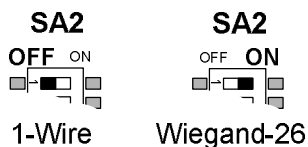
рис. 17. Переключатель SA2.1
