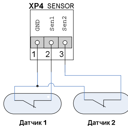
рис. 12. Разъем XP4 (SENSOR) с примером подключения датчиков
