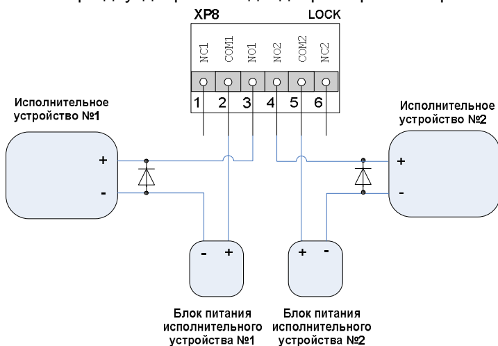
рис. 7. Схема подключения электромеханических замков при двухдверном режиме работы контроллера
