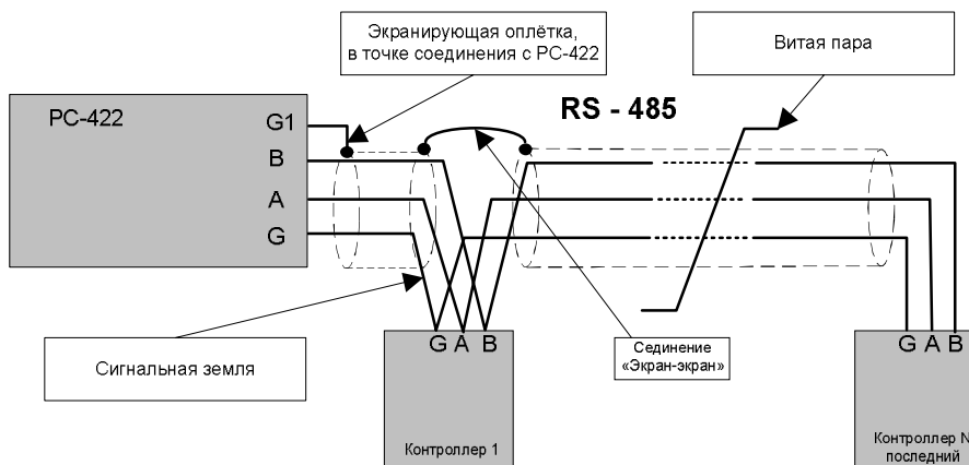
рис. 24. Монтаж линии связи интерфейса RS-485
