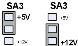
рис. 18. Положение переключки (джампера) SA3
