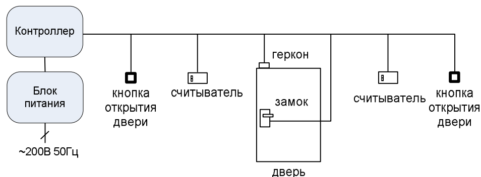
рис. 3. Однодверный режим работы
