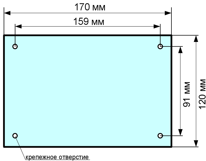
рис. 5. Установочные размеры контроллера
