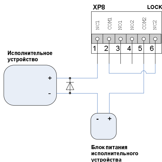
рис. 10. Схема подключения электромагнитных замков при однодверном режиме работы контроллера через контакты обоих реле
