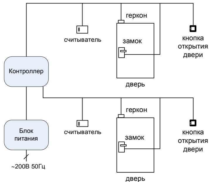
рис. 2. Двухдверный режим работы
