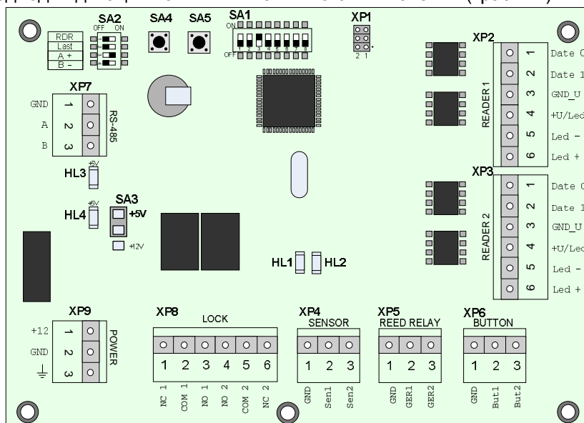
рис. 1. Внешний вид контроллера
