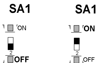
рис. 11. Установка типа конфигурации контроллера
