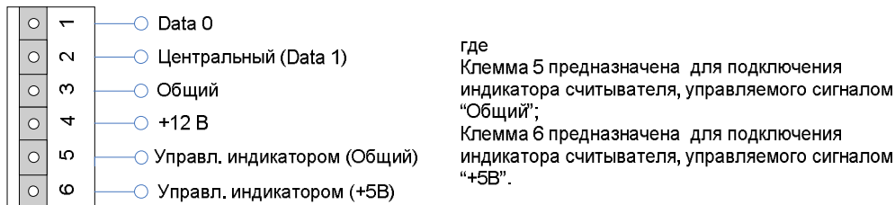
рис. 15. Схема подключения считывателей типа «Wiegand-26» к клеммам XP2 и/или XP3
