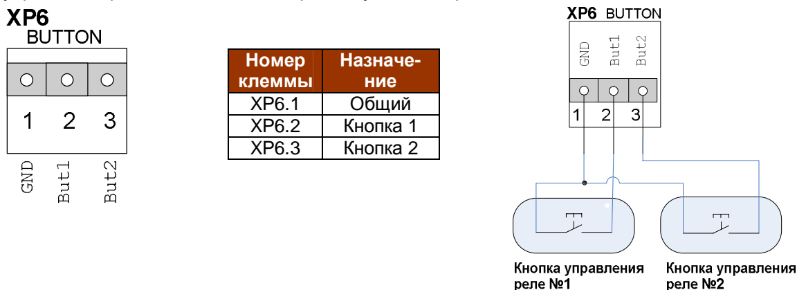
рис. 14. Разъем XP6 (BUTTON) с примером подключения кнопок управления реле
