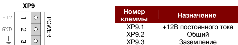
рис. 21. Разъем XP9 (POWER)
