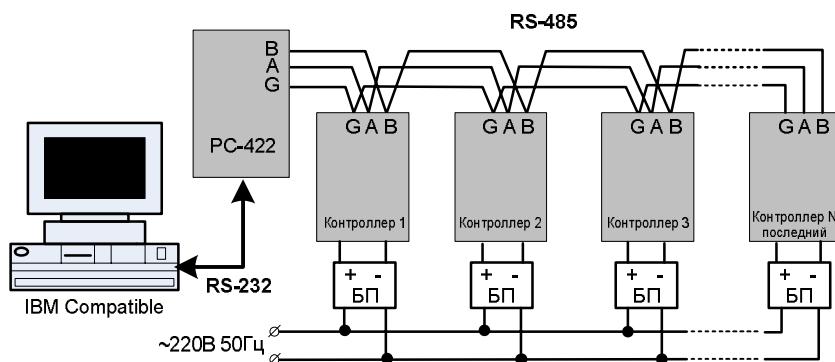
рис. 22. Подключение контроллеров к компьютеру 1
