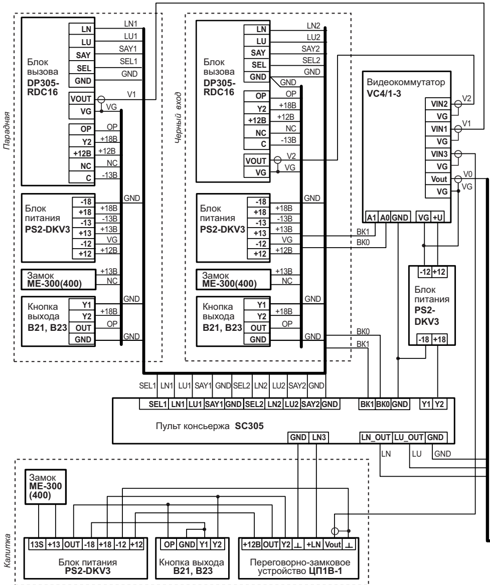
Рис.26 Схема подключения пульта консьержа SC305-D1 (D2)
