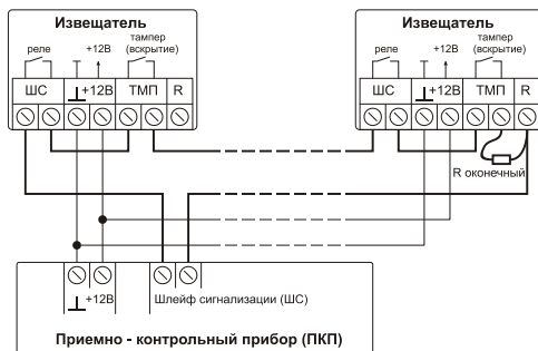
Рис. 4 Схема подключения извещателя
