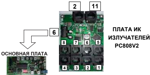
излучающий модуль
