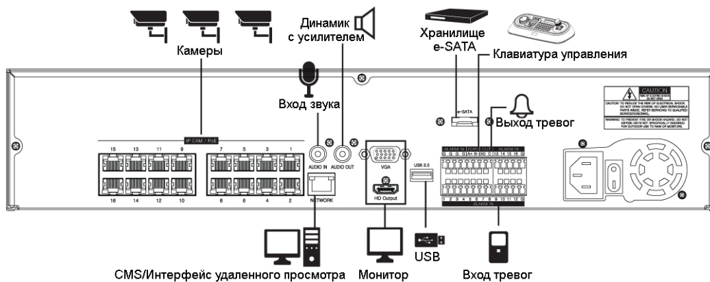
Рис. 2-1 Порядок подключения
