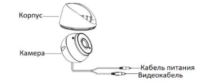
Рисунок 1-16 Камера «шар» II типа
