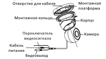
Рисунок 1-18 Камера «шар» IV типа
