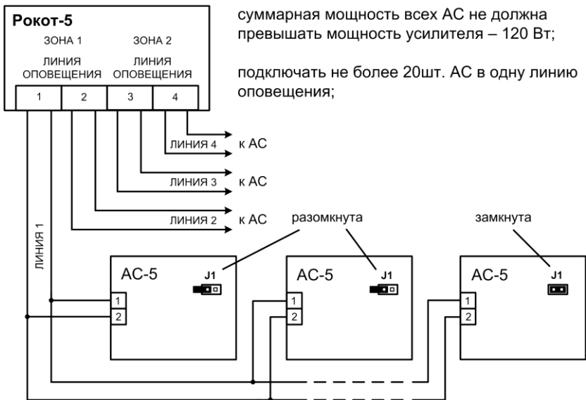
Рис.4б Схема подключений AC-5 к линиям оповещения
