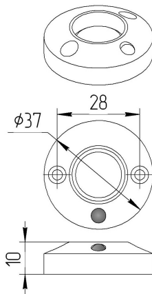
Рис.2 Контакторы КТН, КТН+, КТН-ТК
