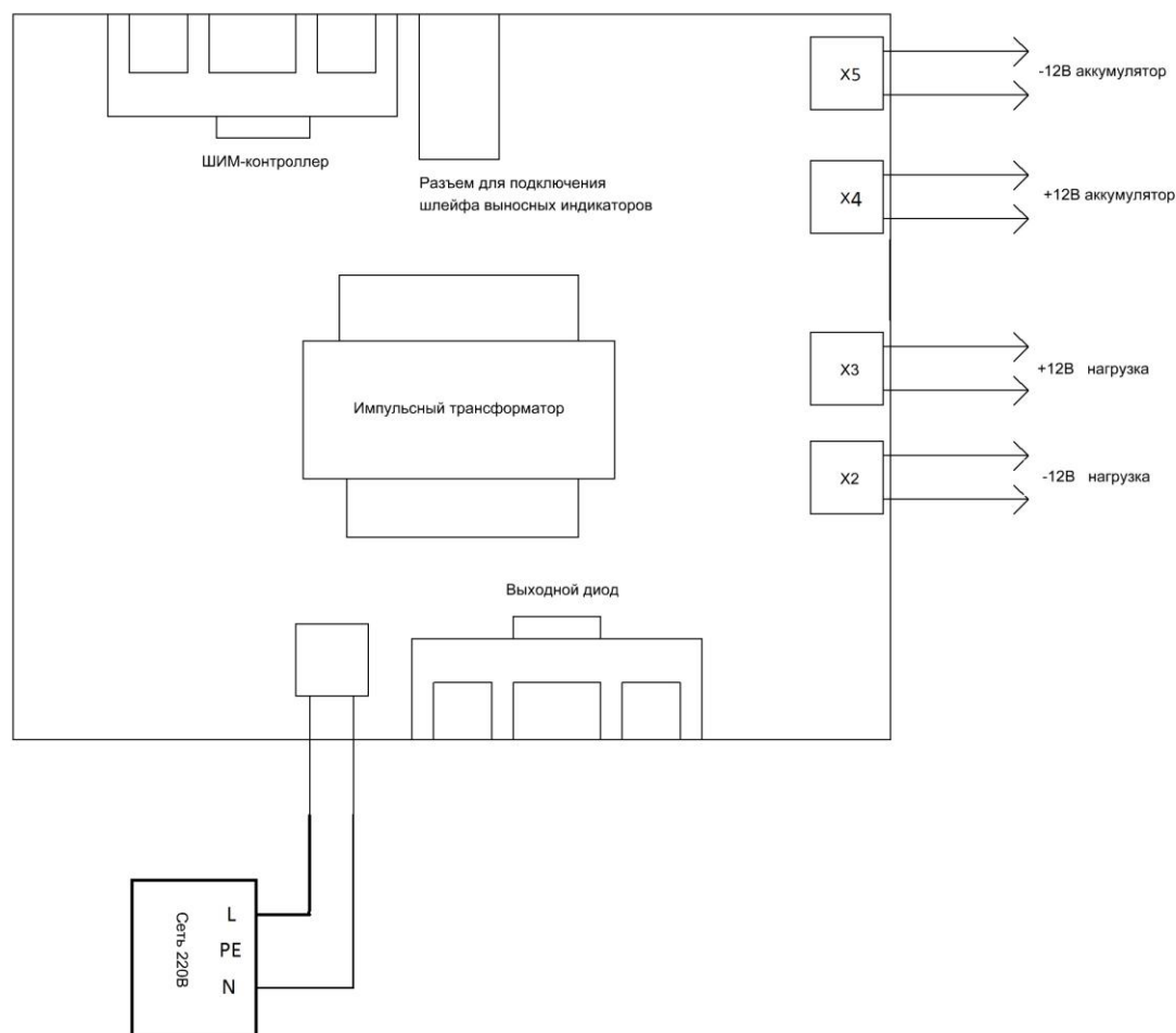
Рис. 1 Схема подключения
