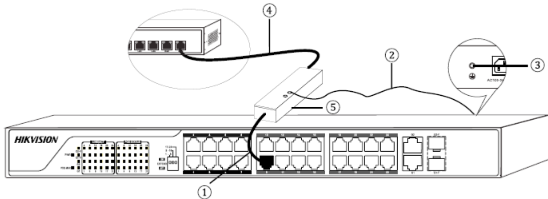
Рисунок 3.4 Подключение молниеотвода
