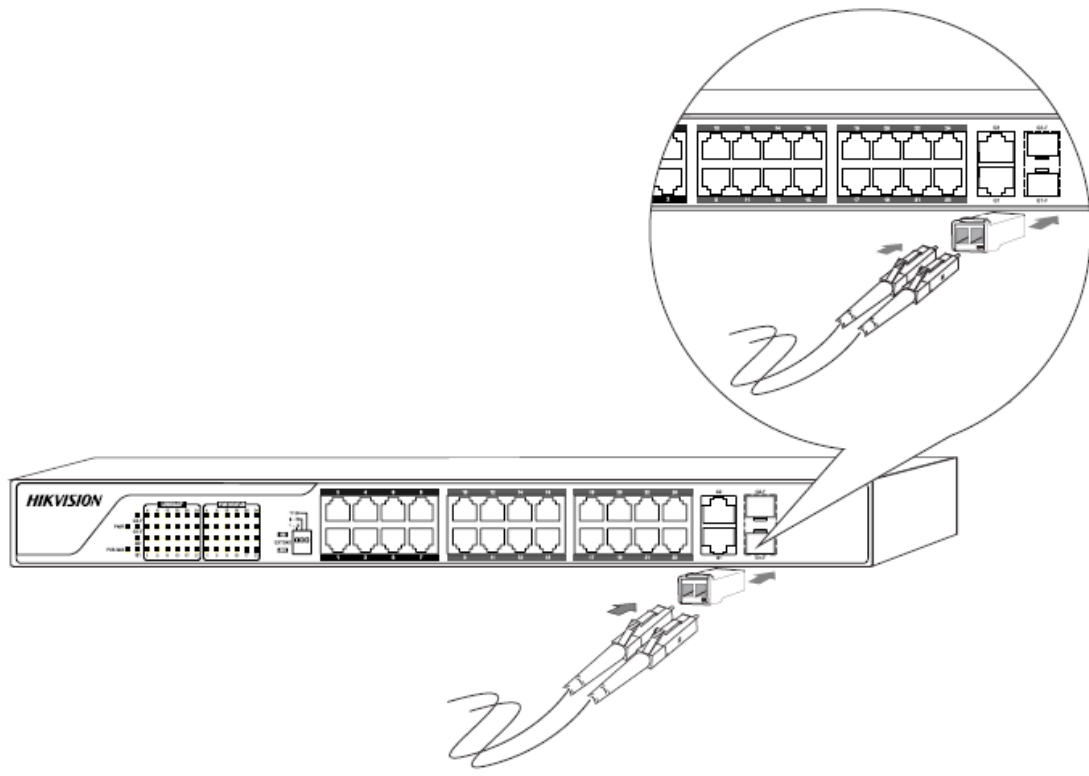
Рисунок 3.3 Установка оптоволоконного кабеля
