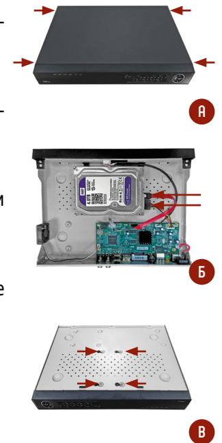
Рис. 1 Установка жесткого диска для моделей в металлическом корпусе
