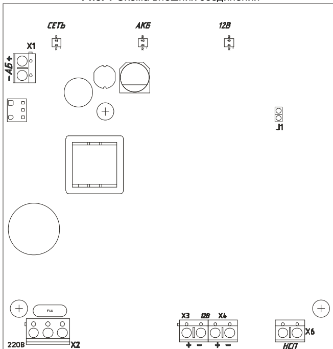
Рис. 1 Схема внешних соединений
