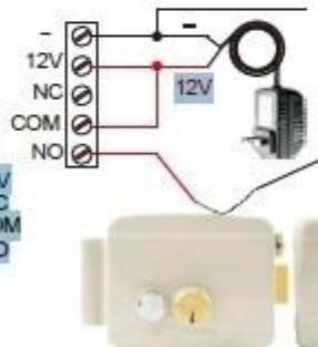
подключение контроллера
