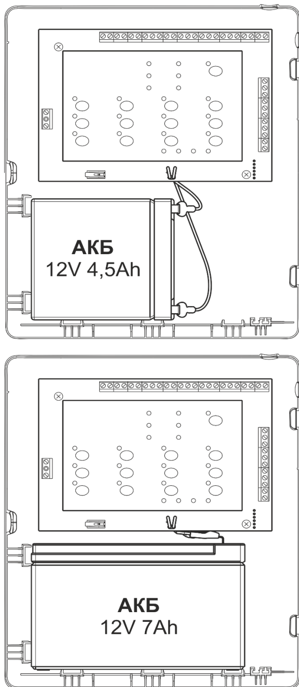
Рис. 9. Расположение в приборе аккумулятора с емкостью 4,5 АЧ и 7 АЧ
