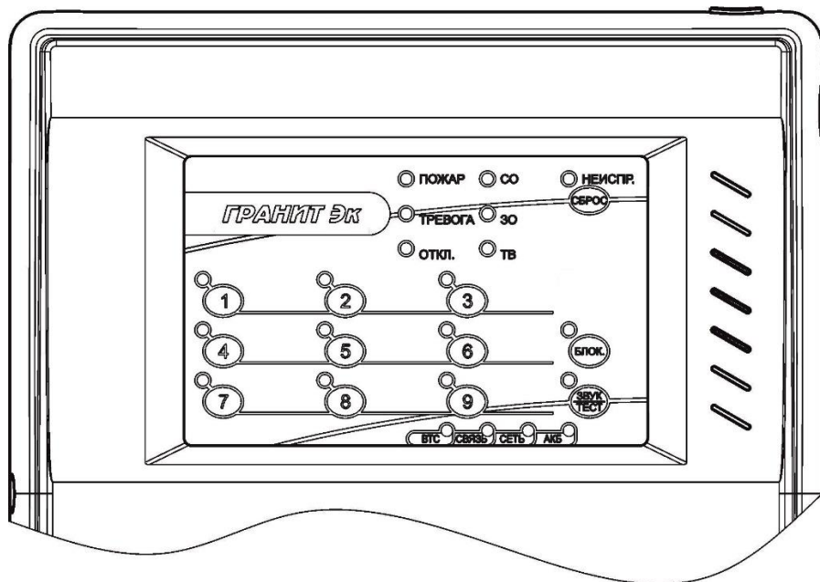
Рис.1. Внешний вид передней панели приборов «Гранит-3 Эк», «Гранит-6ЭК», «Гранит-9 Эк»
