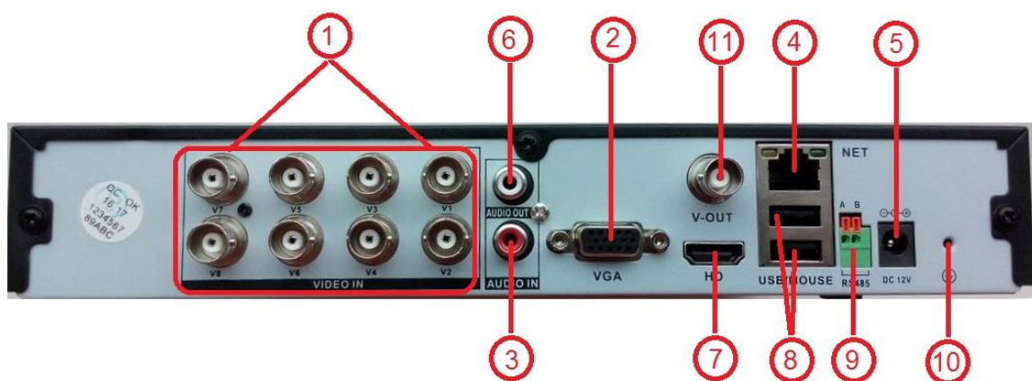
Задняя панель CTV-HD928H Lite
