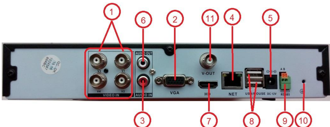
Задняя панель CTV-HD924H Lite
