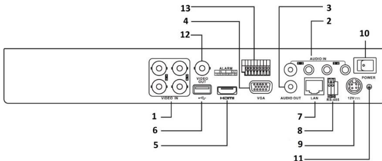
Рисунок 1.4 Задняя панель 2
