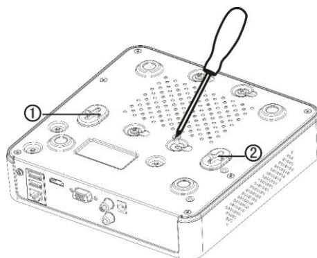
Рисунок 2.2 Крепление HDD
