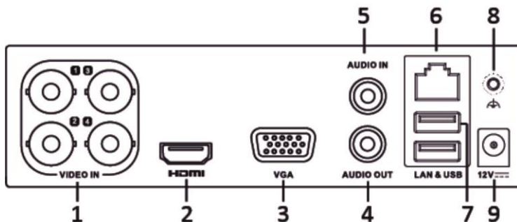
Рисунок 1.3 Задняя панель 1
