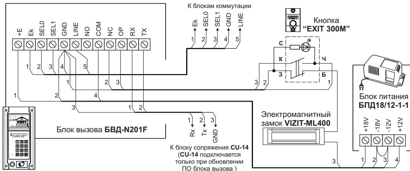
Рисунок 7 - Схема соединений блока вызова БВД-N201F с электромагнитным замком VIZIT-ML400, блоком питания БПД18/12-1-1 и кнопкой "EXIT 300M"
