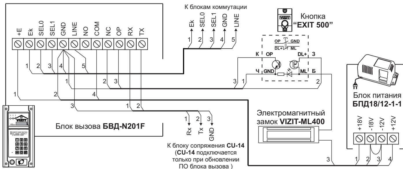
Рисунок 8 - Схема соединений блока вызова БВД-N201F с электромагнитным замком VIZIT-ML400, блоком питания БПД18/12-1-1 и кнопкой "EXIT 500"
