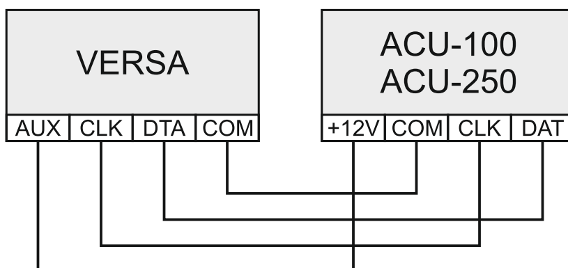
Рис. 12. Способ подключения контроллера ACU-100 / ACU-250 к прибору.
