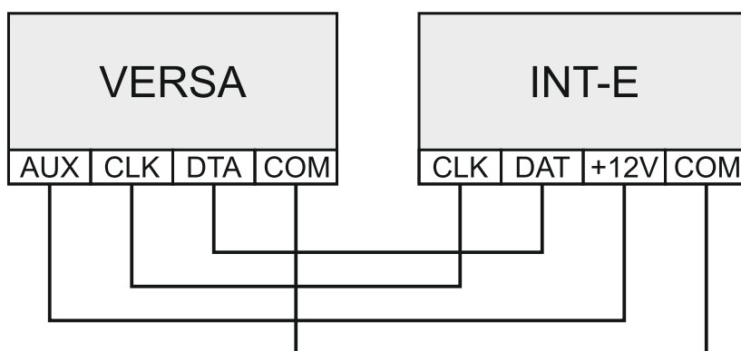
Рис. 15. Способ подключения модуля расширения INT-E к прибору.
