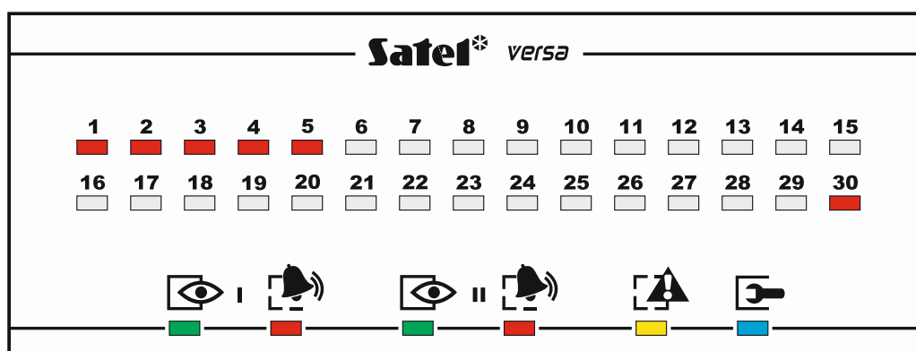
Рис. 27. Настройка адреса светодиодной клавиатуры. Для отображения адреса используются светодиоды с цифрами от 1 до 5 и 30 (адрес 0). Светодиод, отвечающий установленному адресу, быстро мигает, а остальные светодиоды горят.
