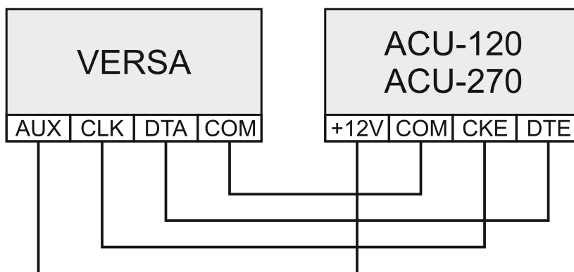
Рис. 11. Способ подключения контроллера ACU-120 / ACU-270 к прибору.
