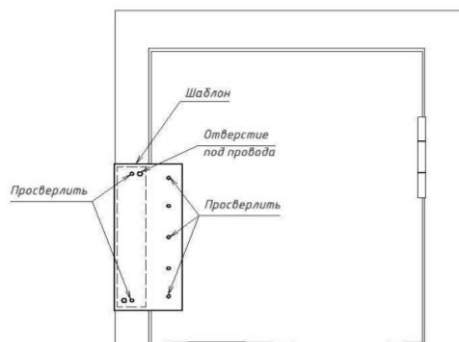
Рисунок 3 – Установка замка по шаблону
