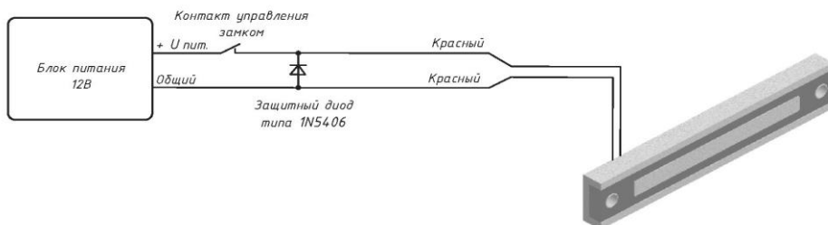
Рисунок 5 – Схема подключения замка ALM-250FT-12
