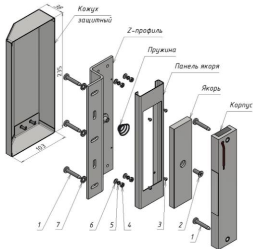
Рисунок 1 – Комплект поставки замка ALM-250FT
