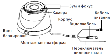
Рисунок 1-22 Камера «шар» VI типа
