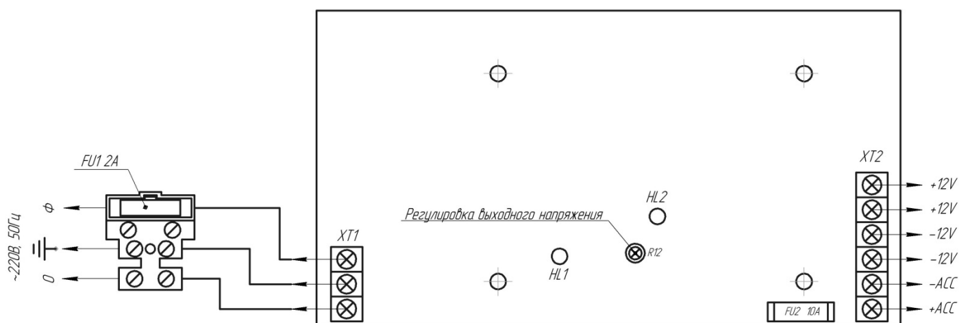
Рис. 1 Схема подключения
