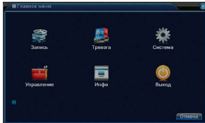
Рисунок 3.3 Главное меню
