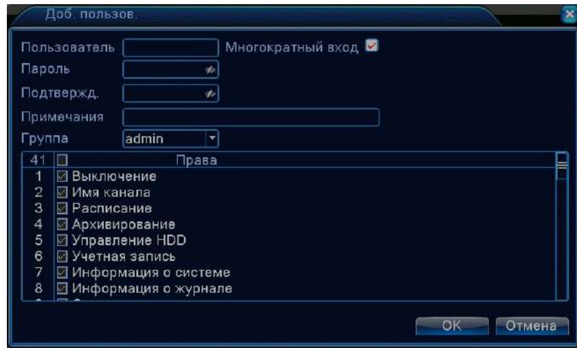
Рисунок 4.47 Добавить пользователя
