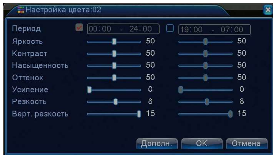
Рисунок 3.18 Настройка цвета
