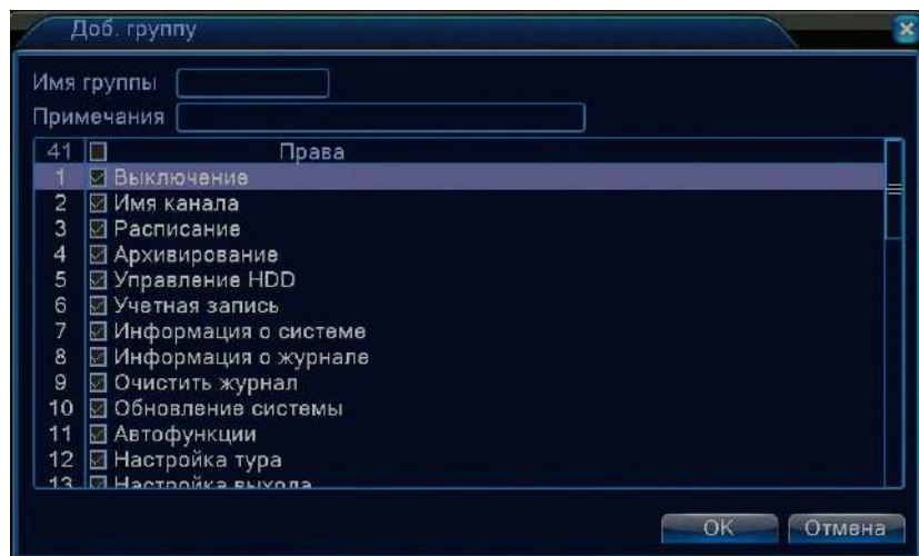
Рисунок 4.48 Добавить группу
