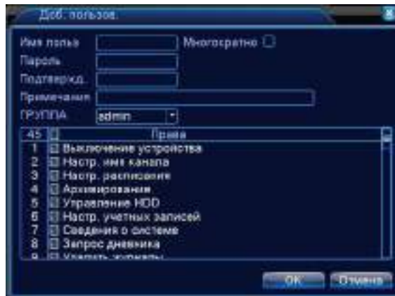
Рисунок 4.43 Добавить пользователя
