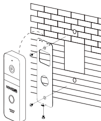
Рис. 4 Фронтальная установки видеопанели
