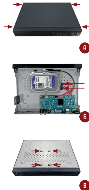
Рис. 3 Установка жесткого диска для FR1104 | FR1108 | FR1204 | FR1208 | FR2116 | FR2216
