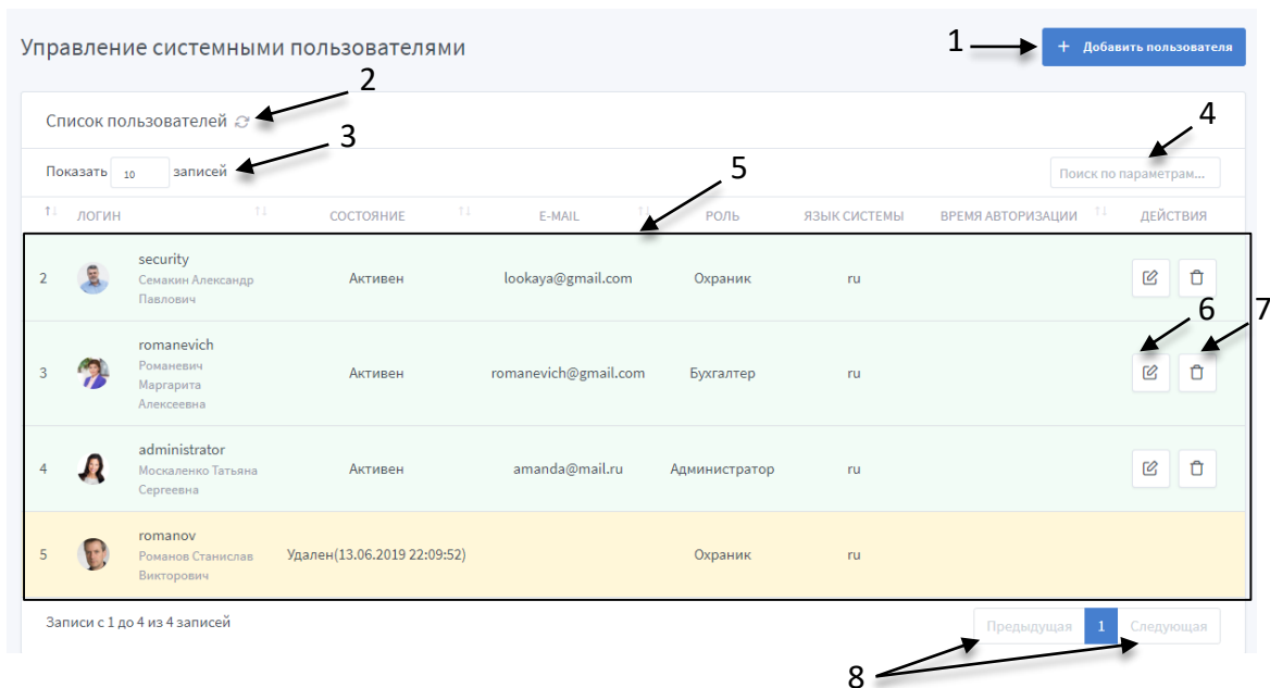
Рис. 79 Пользователи системы
