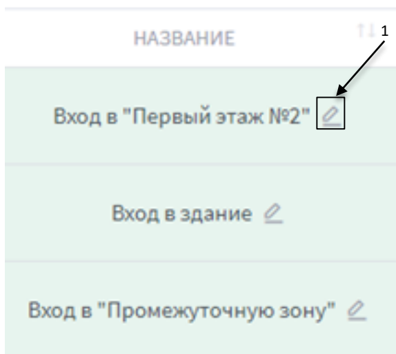
Рис. 39 Добавление названия
