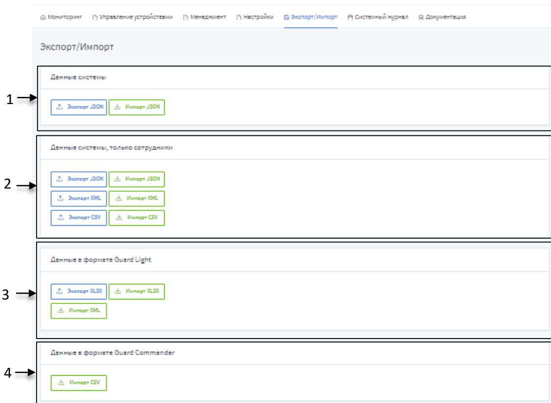
Рис. 75 Страница "Экспорт/Импорт"
