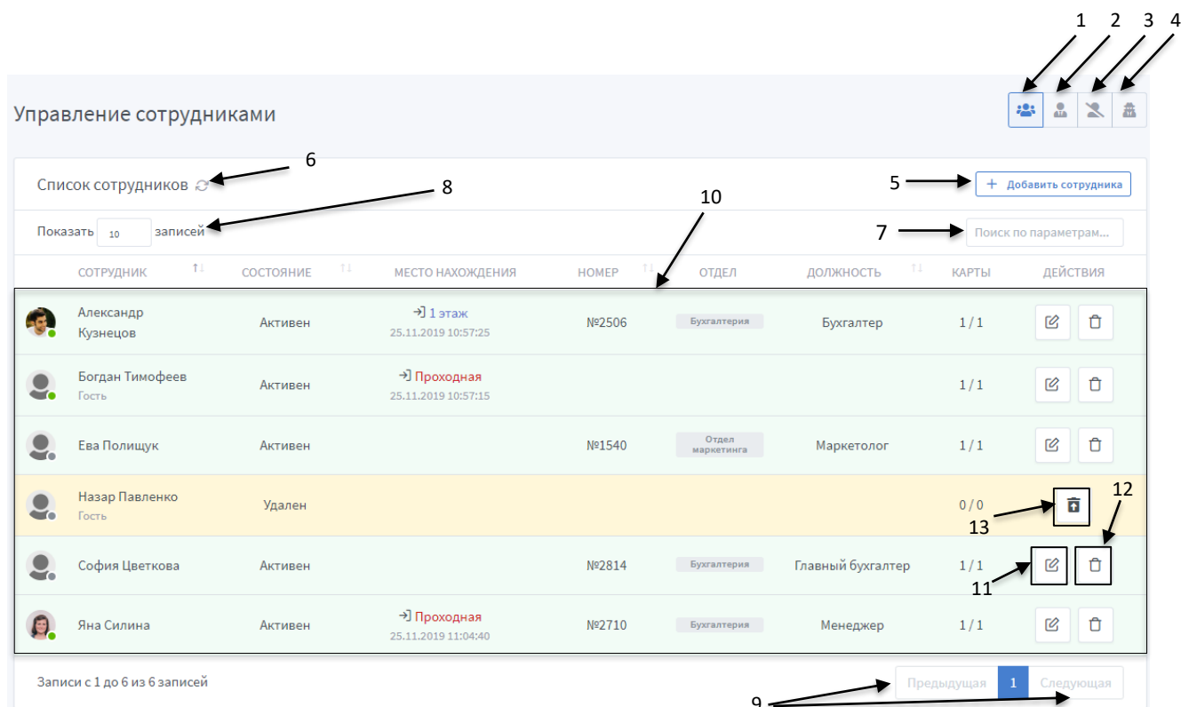
Рис. 46 Страница «Сотрудники»
