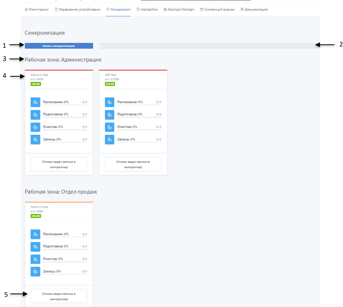
Рис. 69 Страница "Синхронизация"
