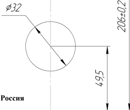
Рис.1. Разметка под установку блока вызова
