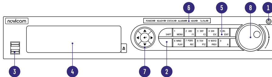
Рис. 9 Пример интерфейса передней панели NR4832
