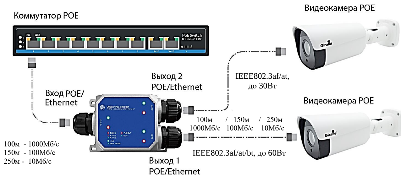
Рис. 4. Подключение устройств к Изделию
