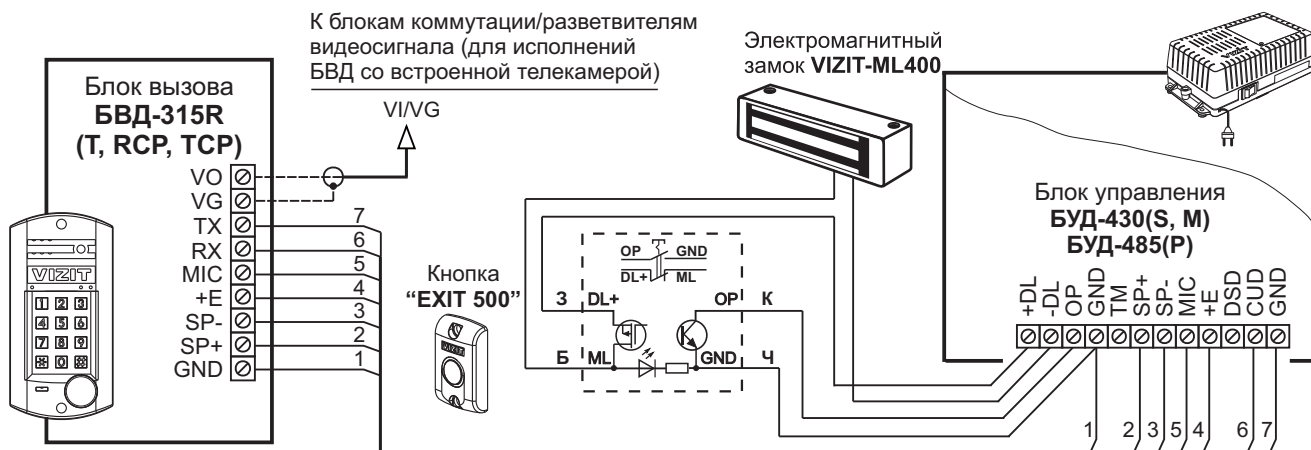
Рисунок 10 - Схема соединений блока вызова БВД-315R(Т, RCP, TCP) с блоком управления БУД-430(S, М), БУД-485(P) , электромагнитным замком VIZIT-ML400 и кнопкой “EXIT 500”
