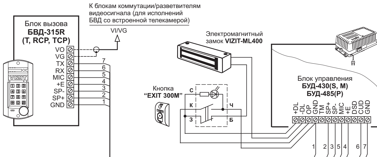
Рисунок 9 - Схема соединений блока вызова БВД-315R(Т, RCP, TCP) с блоком управления БУД-430(S, М), БУД-485(P) , электромагнитным замком VIZIT-ML400 и кнопкой EXIT 300M
