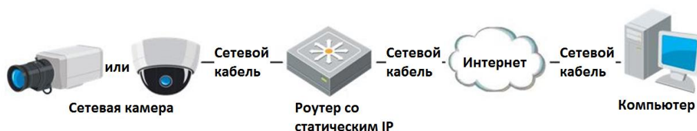
Рисунок 2-10 Доступ к видеокамере через роутер со статическим IP-адресом
