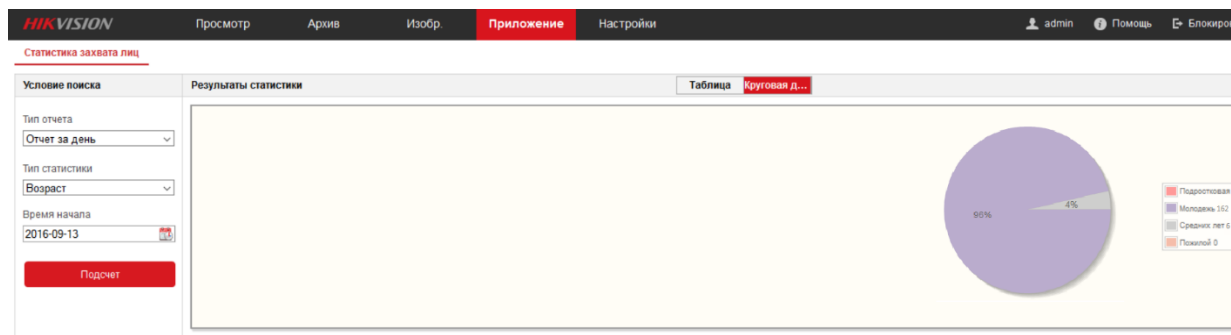
Рисунок 14-1 Интерфейс Приложение
