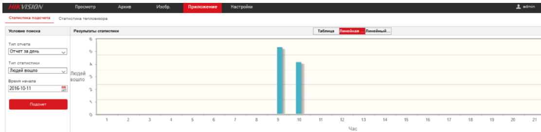
Рисунок 14-2 Подсчет людей
