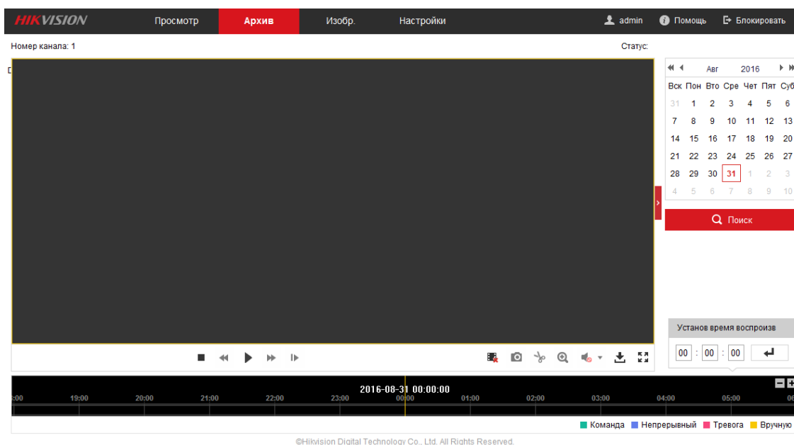
Рисунок 12-1 Интерфейс воспроизведения
