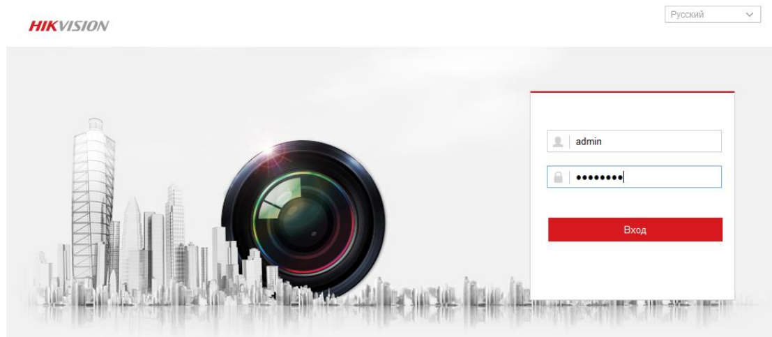
Рисунок 3-1 Интерфейс авторизации
