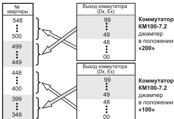
Рис.3 Пример схемы подключения двухсот квартир к двум коммутаторам КМ100-7.2
