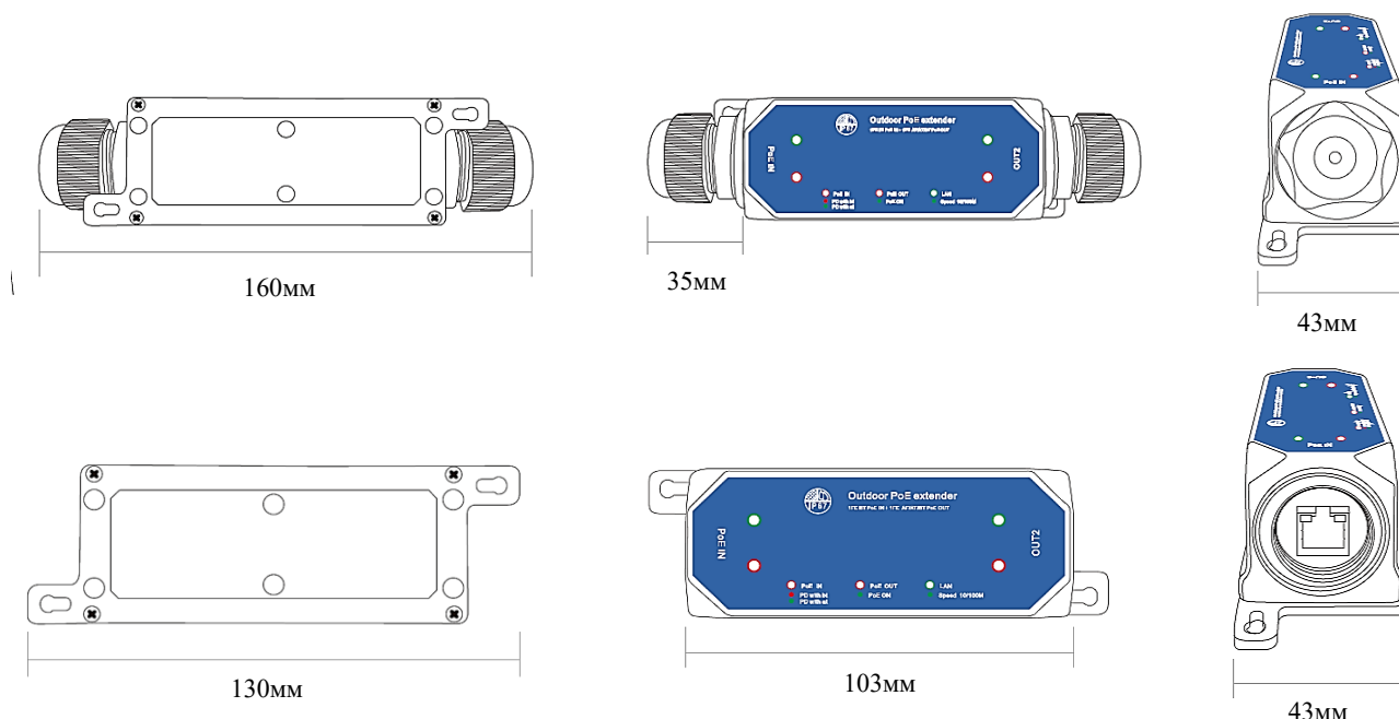
Рис. 1. Габаритные размеры
