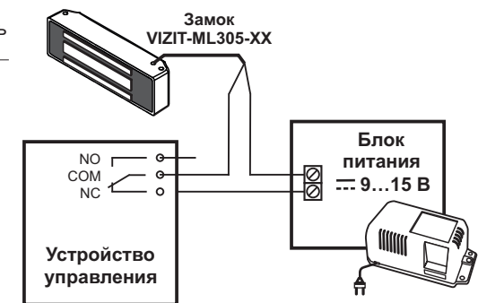
Рисунок 4 - Схема включения замка
