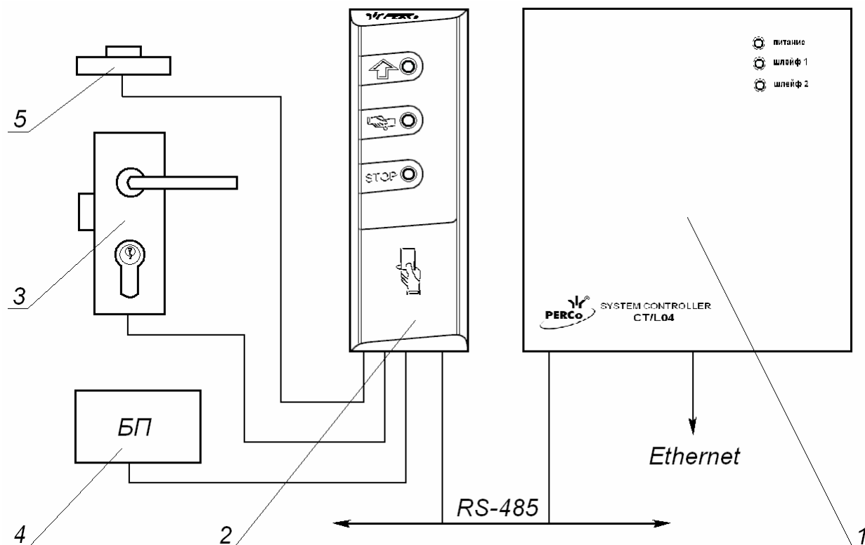
Рисунок 1. Функциональная схема
